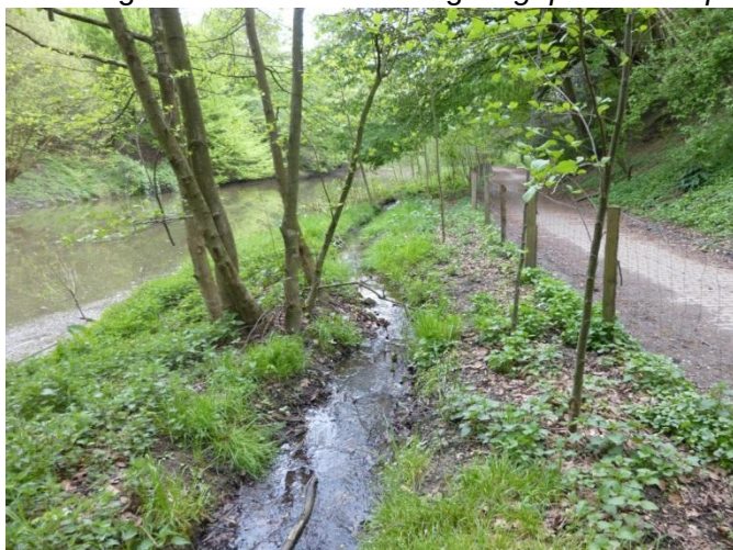
Abbildung 4.20: Probestelle Hor1
