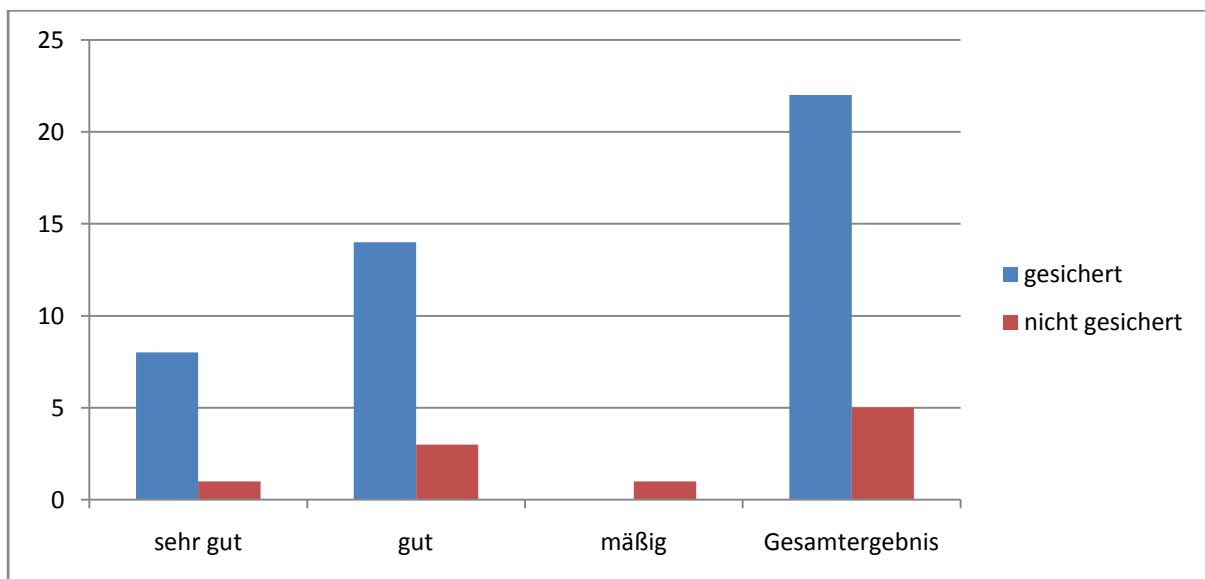
Abbildung 3.9: Verteilung Saprobie
