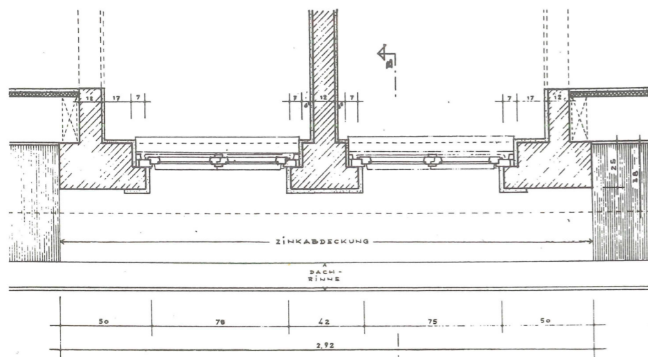
HAUSTYP F : DACHGAUBE ANSICHT - VERTIKALSCHNITT HORIZONTALSCHNITT
