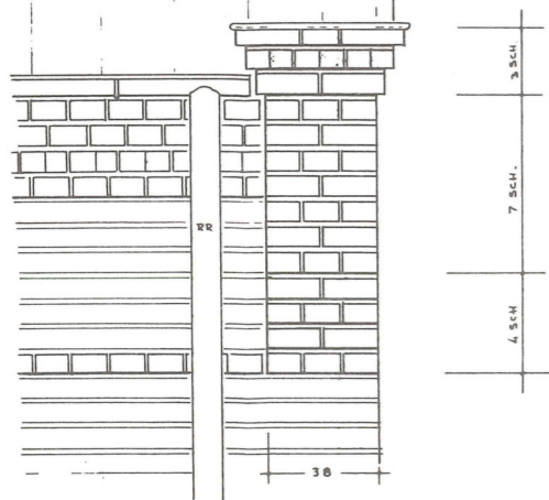
HAUSTYP A,G : GIEBELOHR SEITENANSICHT - VORDERANSICHT
