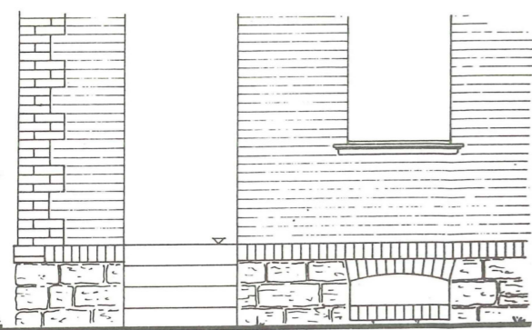
HAUSTYP A,G : GIEBELOHR SEITENANSICHT - VORDERANSICHT
