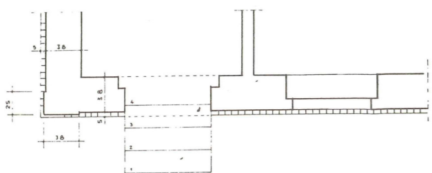
HAUSTYP A,B: BRUCHSTEINSOCKEL
