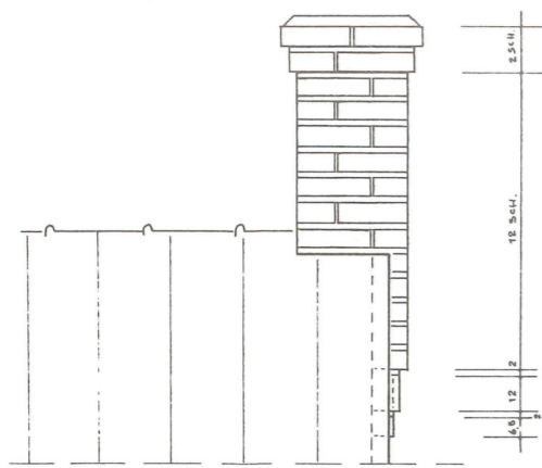
HAUSTYP A,G : KAMINKOPF SEITENANSICHT - VORDERANSICHT
